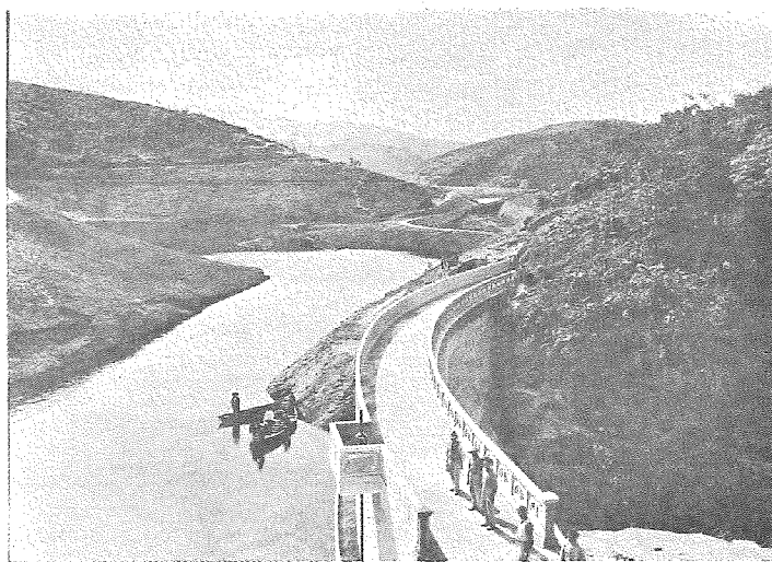
Foto da barragem do Cabuçu, a primeira grande obra de concreto do Brasil, feita no período de 1905 a 1907, com cimento vindo da Inglaterra.
